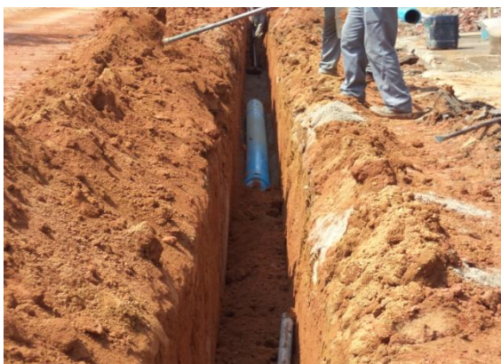
Foto 01: assentamento da rede de 200mm FoFo e rede 50mm de PVC – PBA.
