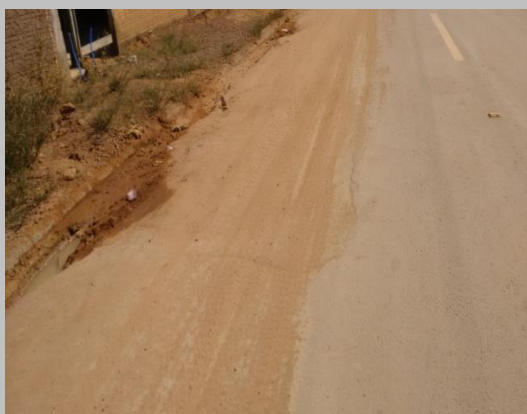
FOTO 03: rachaduras e afundamento local comprometimento da base.
